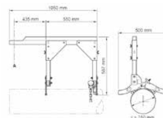
Dispositivo di taglio a sbalzo
