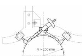
Dispositivo per tubi di piccolo diametro
