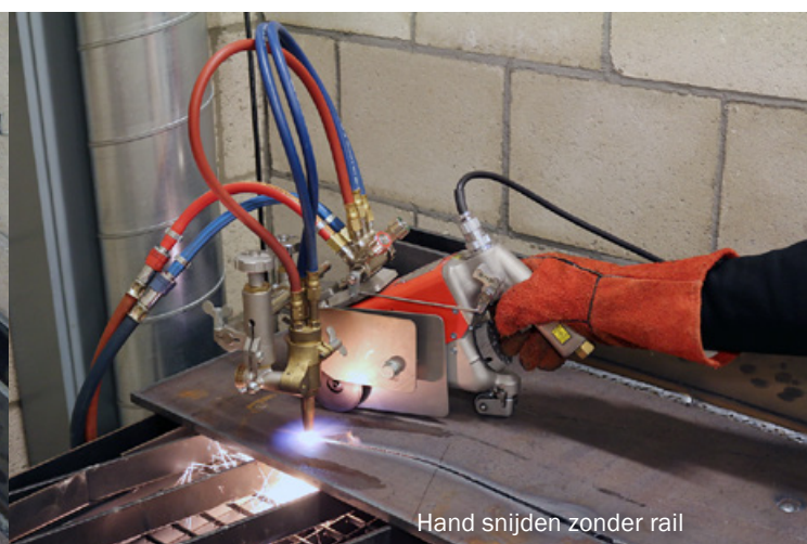
Recht snijden met IK-93 rail
