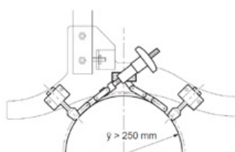
Hulpstuk voor kleine pijp- \varnothing
