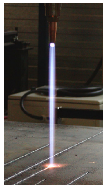
KOIKE high speed D nozzle gemaakt voor de beste snijkwaliteit. Test bij Koike op 275 mm hoogte vanaf de plaat. Nozzle: 106-D7#0.
