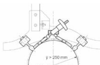
Support de tube petit diamètre
