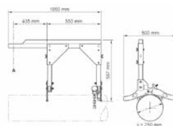
Support de coupe suspendu
